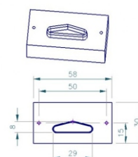
Driehoekige pons
