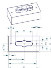
Symetrische pons
