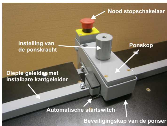
Details van de ponskop met automatische startswitch
