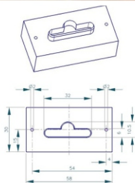
Standaard pons
